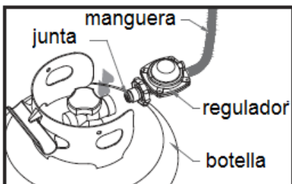
Conexión manguera / regulador y conexión regulador / botella
